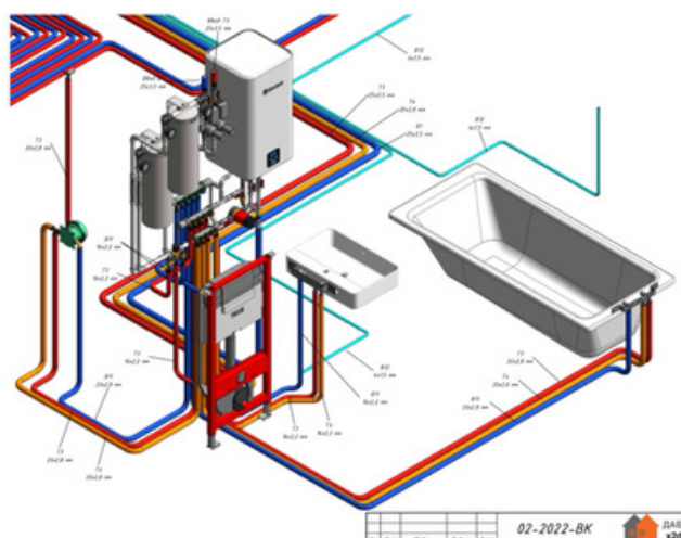
АксонOMETрическая схема водоснабжения
