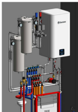
Санузел. Узел ввода воды.
