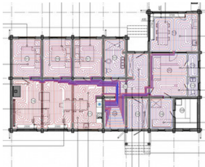
План этажа. Теплый пол
