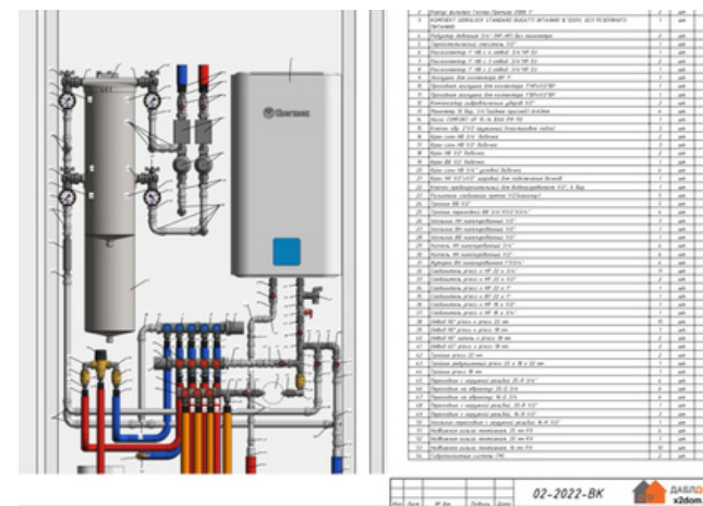
Узел ввода. Спецификация узла ввода.
