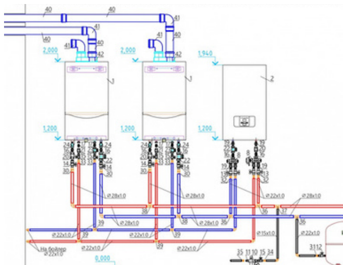
Монтажная схема обвязки котельной
