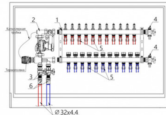
Монтажная схема коллектора теплого пола
